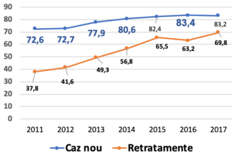
TB sensibilă
