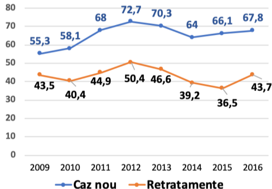
TB MDR
